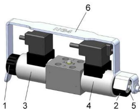
Wegeventil NG4
