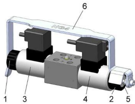
Wegeventil NG4
