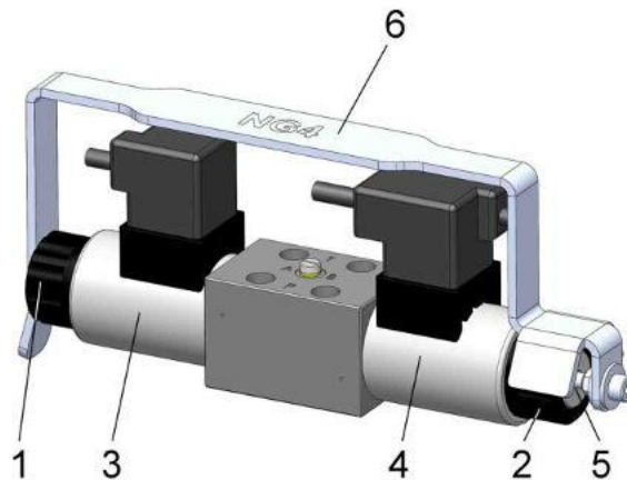
Beispiel: Wegeventil NG4
