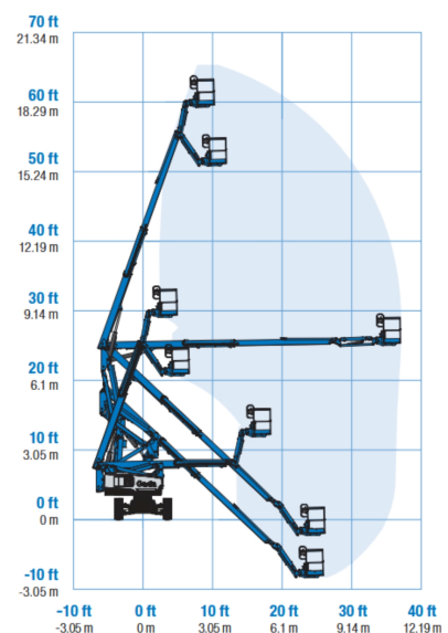
Gelenkteleskop GTB 200 "Maik" Genie Z-60 FE
