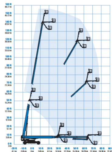
Arbeitsdiagramm SX-150
