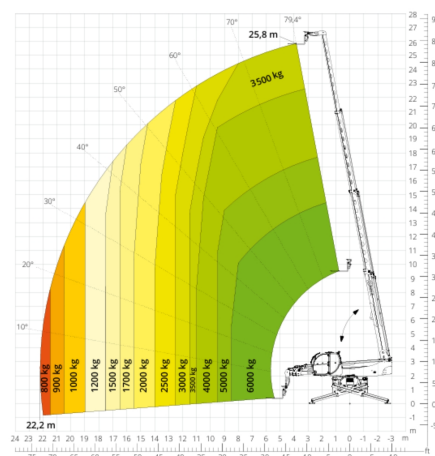
Lastdiagramm mit AUSGEFAHRENEN STÜTZEN 360° ATT-03-004
