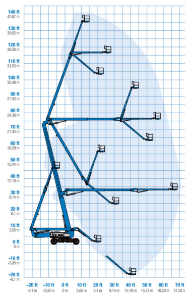
Gelenkteleskop GTB 430 Genie ZX-135/70
