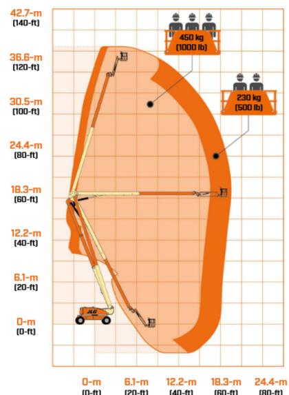
Gelenkteleskop GTB 400 JLG 1250AJP
