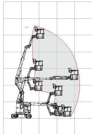
Gelenkteleskop-Arbeitsbühne GTB 120 Sinoboom AB 10ERJN
