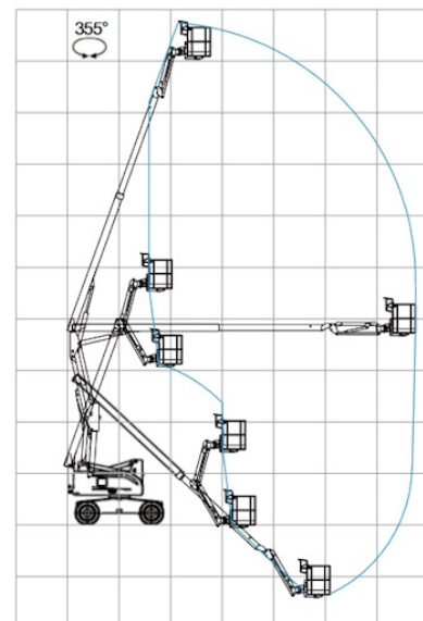
Gelenkteleskop GTB 200 Sinoboom AB18EJ "Michel"
