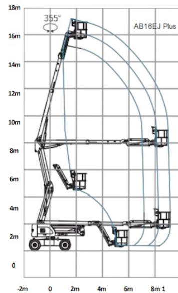
Gelenkteleskop GTB 180 Sinoboom AB16EJ Plus "Fritz"
