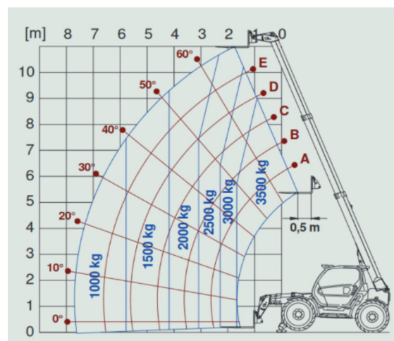
Teleskopplader TS 120M Merlo P35.11
