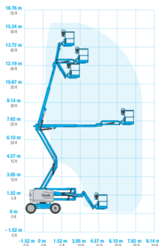
Arbeitsdiagramm Z-45/25J RT
