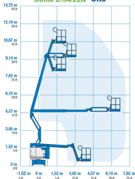
Gelenkteleskop GTB 120 Genie Z-34/22N "Otto"
